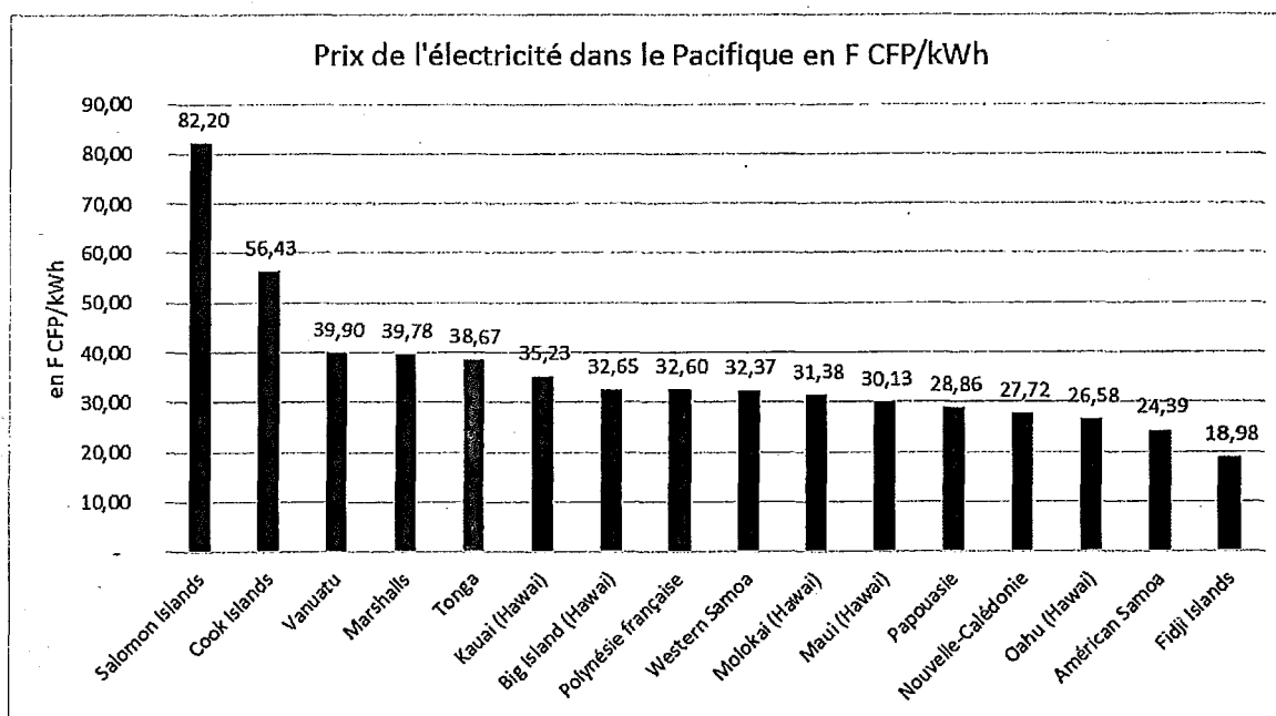
Graphique n° 6 : Prix moyen de l'électricité dans les pays du Pacifique, en F CFP/kWh :
