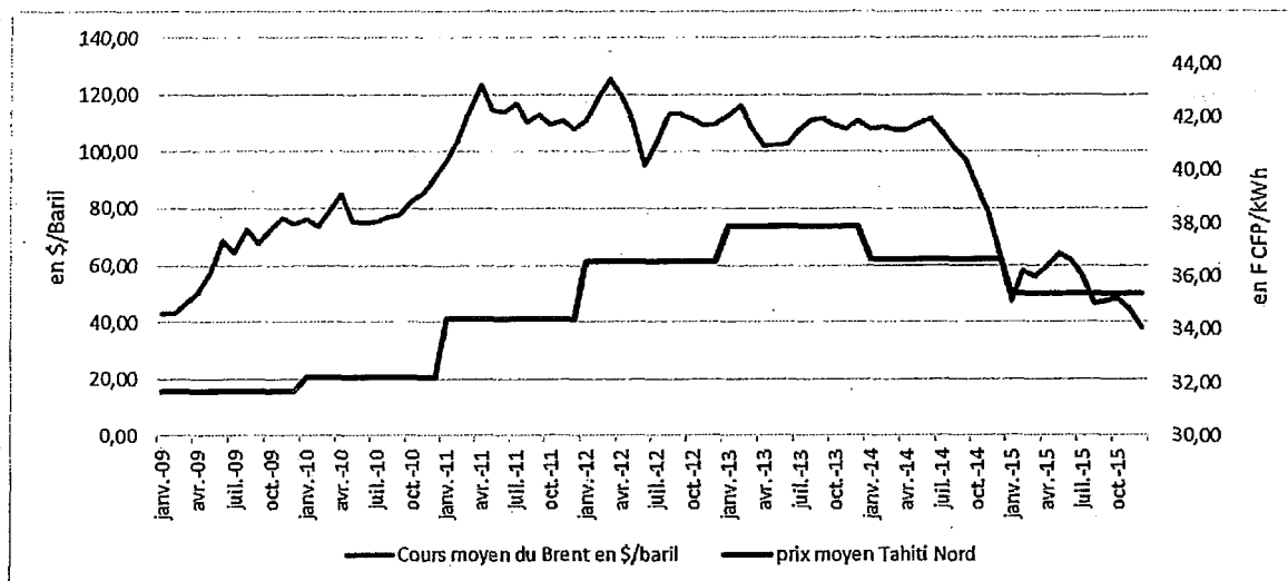
Graphique n° 8 : Evolution du cours du pétrole, en $/baril, et du prix de vente moyen sur la concession de Tahiti Nord, en F CFP/kWh :
