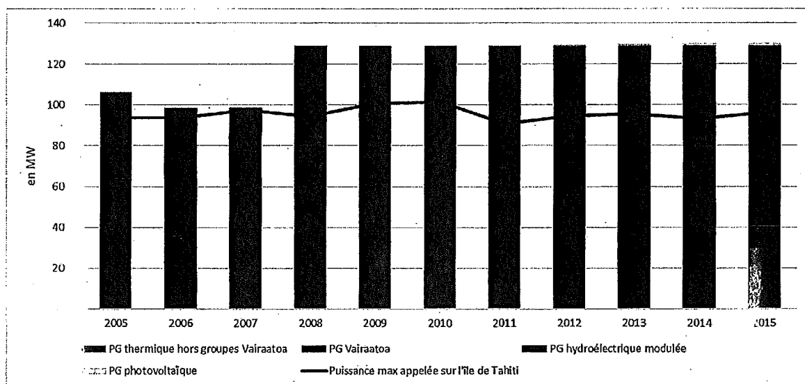
Graphique n° 4 : Puissance garantie de sécurité par type de production entre 2005 et 2015, en MW :
