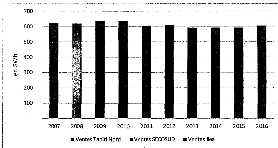
Graphique n° 2 : Ventes d'électricité, Tahiti Nord, SECOSUD et les autres îles, en GWh :
